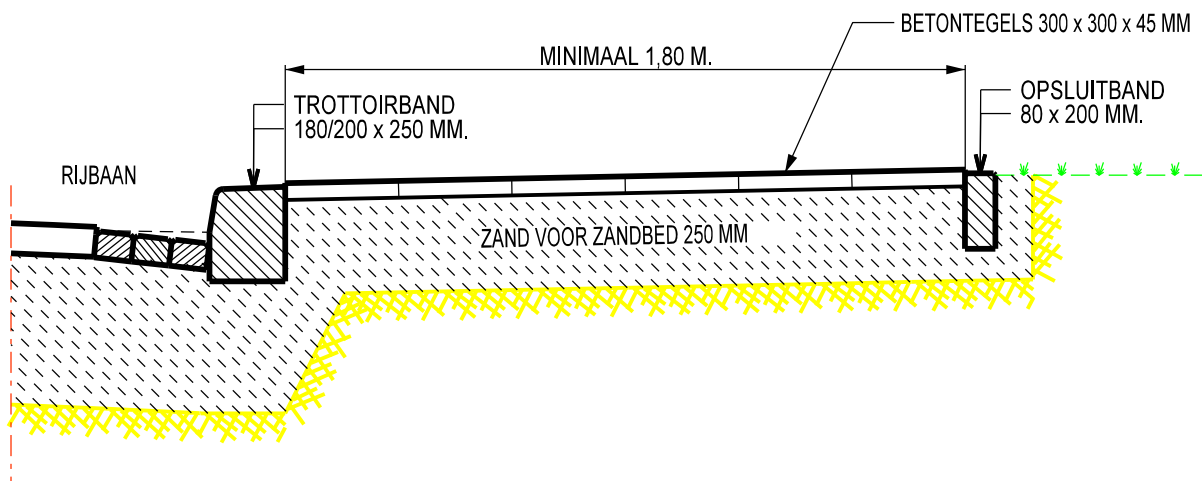
Voetpad aanliggend (elementenverharding)
