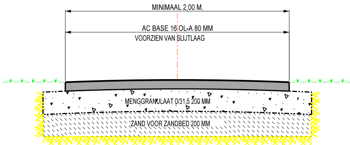
Voetpad vrijliggend (asfalt)
